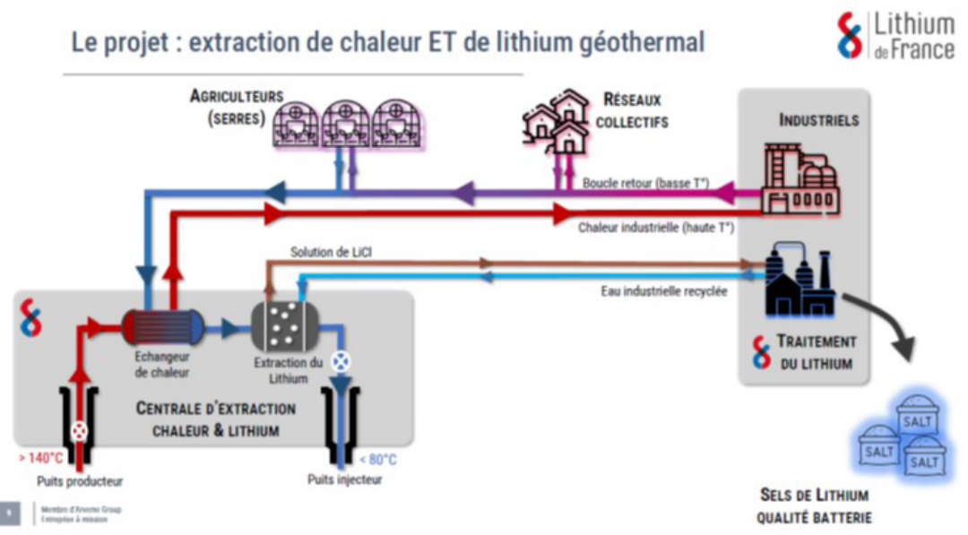
Schéma d'un projet de co-valorisation de la chaleur et du lithium géothermal – Source : Lithium de France (DLE : unité d'extraction directe de lithium)
