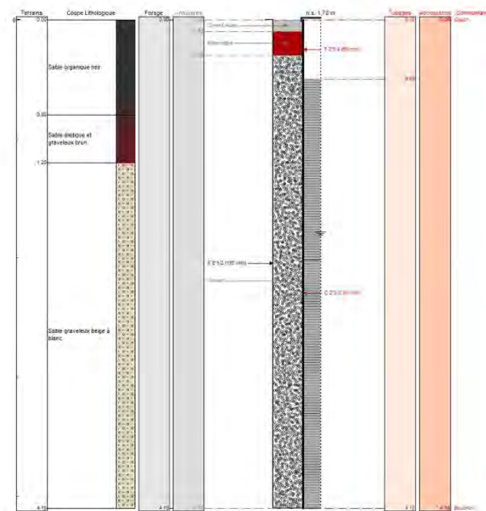
Figure 21 : Coupe lithologique et technique du piézomètre Pz2 (Réalisation : CERAG)
