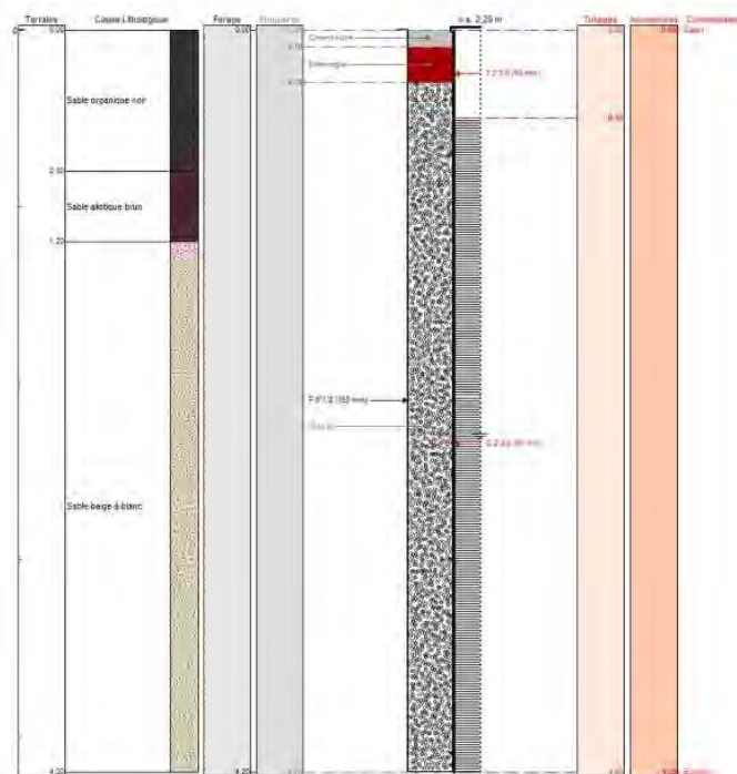
Figure 20 : Coupe lithologique et technique du piézomètre Pz1 (Réalisation : CERAG)
