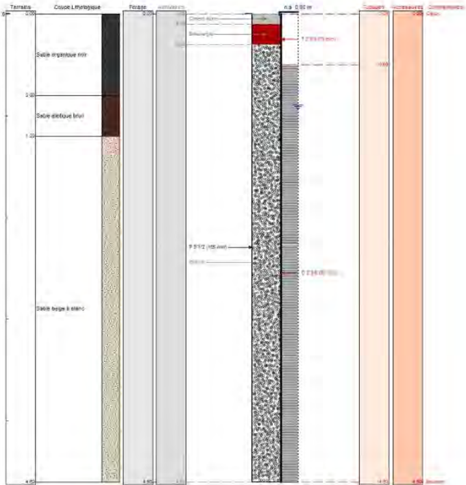
Figure 22 : Coupe lithologique et technique du piézomètre Pz3 (Réalisation : CERAG)
