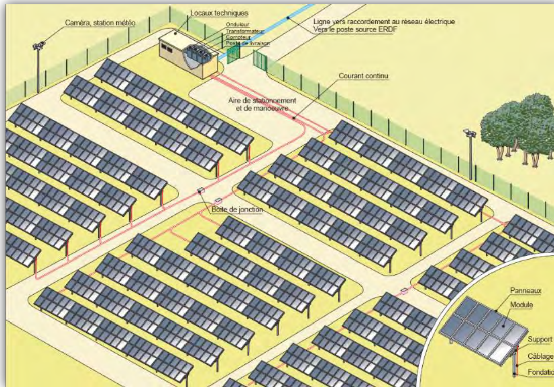
Figure 16 : Principe d'implantation d'une centrale solaire
