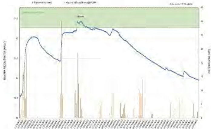
Figure 23 : Suivi du niveau piézométrique en mNGF dans Pz1 et pluviométrie journalière au niveau de la station de Bordeaux-Mérignac (Réalisation : CERAG)
