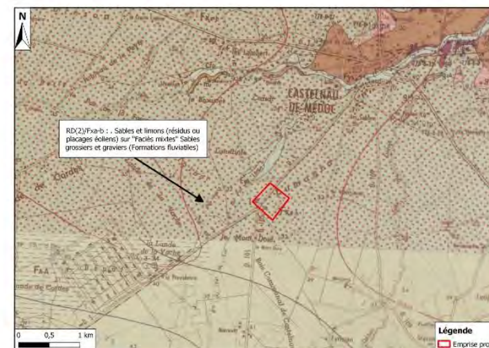
Figure 5 : Extrait de carte géologique au 1/50 000 (Source : BRGM Infoterre ; Réalisation : CERAG)
