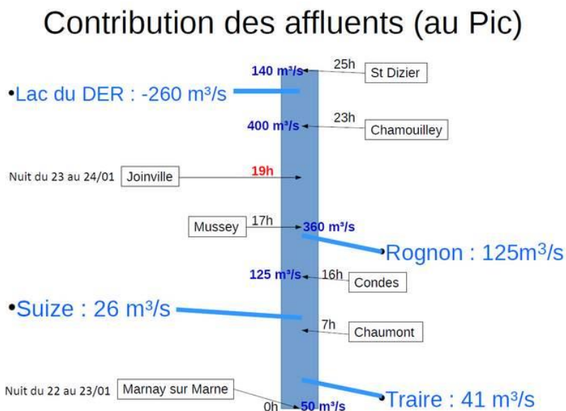
Figure 71 Contribution des affluents au pic de crue de la Marne amont - Source SPC SAMA
