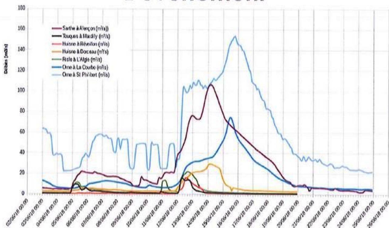
Figure 110 Hydrogramme de crue de l'Orne et de la Risle en juin 2018 – Source DDT 61
