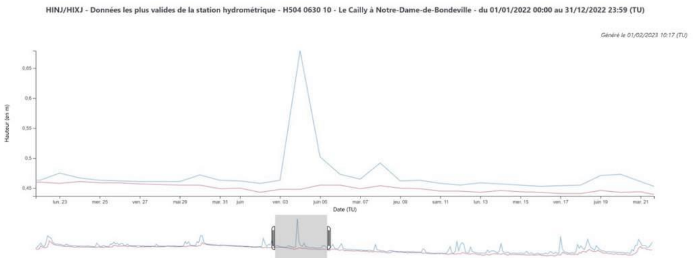
Figure 134 Hydrogramme et pic de crue sur le Cailly - 04/06/2022 - Source DDTM 76
