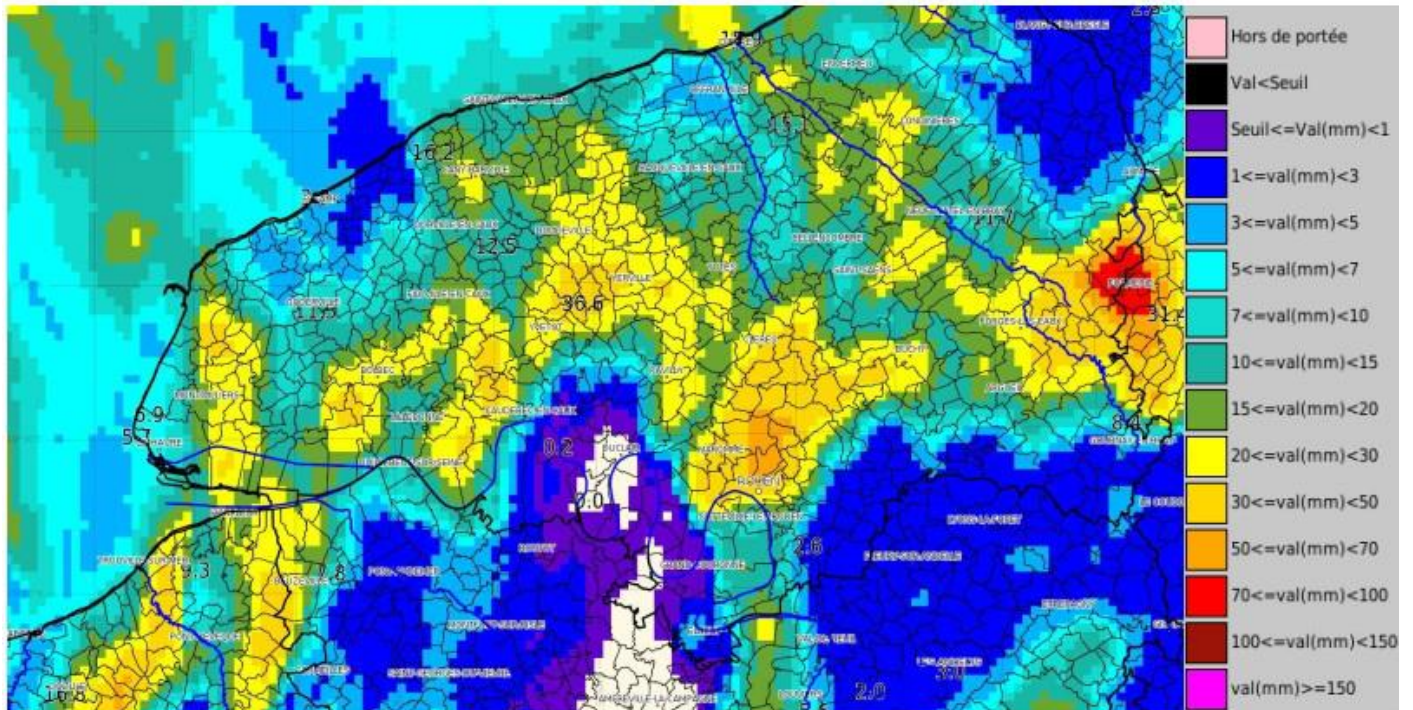
Fig 4 : Lame d'eau Antilope (Fusion Radar/pluviomètre) ré-analysée à J+1 du 4 juin 2022 de 17h00 à 21h00 locales (cumuls sur 4h). La légende est visible sur la droite de la figure. On note des valeurs d'un peu plus de 50 mm sur les communes de Houpeville, Isneauville et Bois-Guillaume. Les valeurs des pluviomètres sont indiqués en noir (cumuls sur 6h, mais il n'a pas plus les 2 premières heures, c'est donc comparable avec la lame d'eau).
