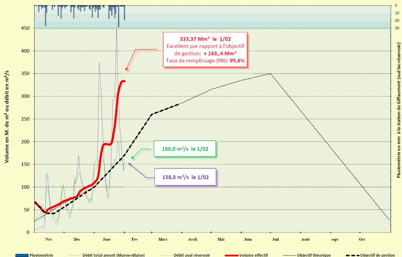
Figure 105 Courbe d'exploitation du lac-réservoir Marne - Source DDT 52
