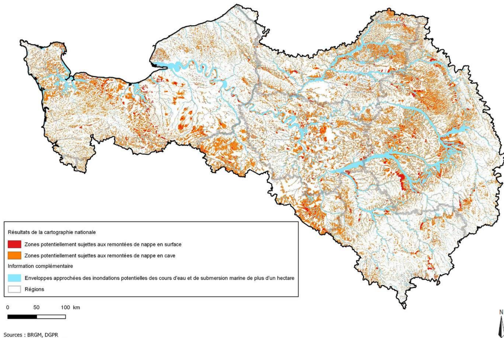
Figure 7 Extrait de la carte nationale de sensibilité aux remontées de nappe - Bassin Seine-Normandie - Source BRGM
