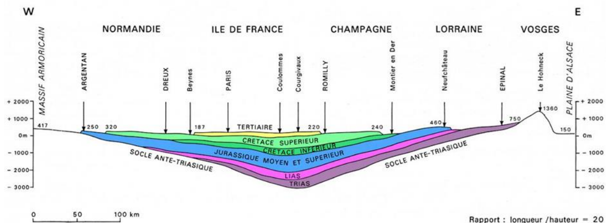
Figure 5 Schéma de la géologie du bassin Seine-Normandie vue en coupe- Source Piren Seine
