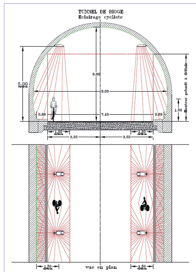
Schéma de principe d'implantation des luminaires spécifiques cyclistes (© CD74)
