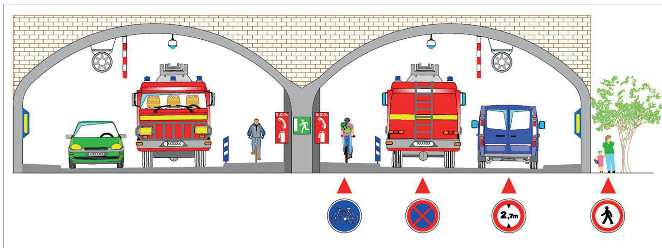
Principe d'aménagement du tunnel Jenner (© CETU)
