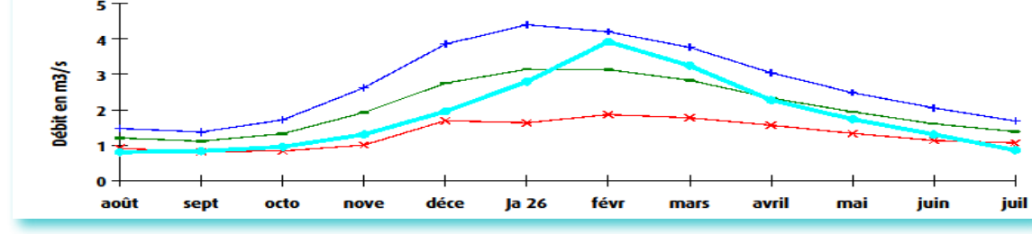
La Canche à Brimeux, représentative des cours d'eau côtiers alimentés par la nappe de la craie. Surface du bassin versant: 894 km². Débit internannuel: 12.10 m³/s
