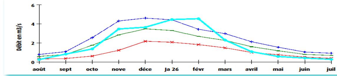
La Liane à Wirwignes, représentative des fleuves côtiers du Boulonnais. Surface du bassin versant: 100 km². Débit internannuel: 1.83 m³/s
