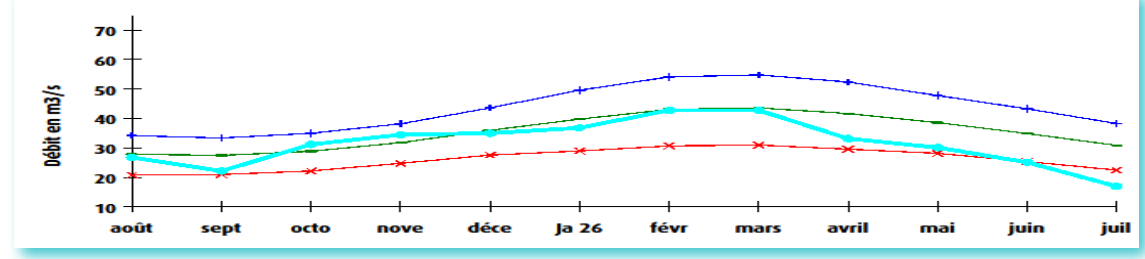
La Somme à Abbeville, représentative des cours d'eau de la Picardie. Surface du bassin versant: 5560 km². Débit internannuel: 35.1 m³/s
