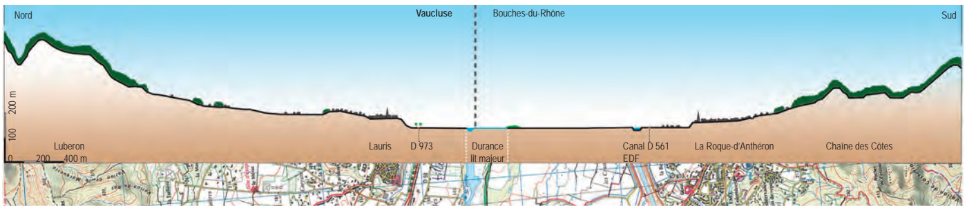
COUPE TOPOGRAPHIQUE - AGENCE PAYSAGES
