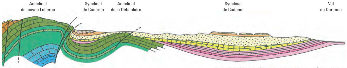
COUPE DE M. LIOUVILLE, GUIDE GÉOLOGIQUE DU LUBERON, PNR LUBERON, ÉDITIONS BRGM, 1998
