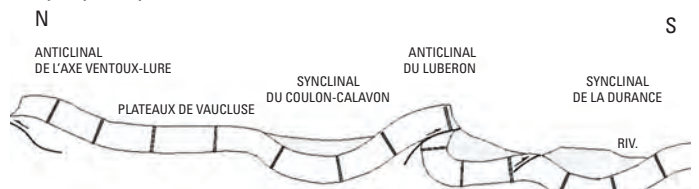
COUPE GÉOLOGIQUE SIMPLIFIÉE DU MONT-VENTOUX À LA DURANCE, GUIDE GÉOLOGIQUE DU LUBERON, BRGM - PNR DU LUBERON
