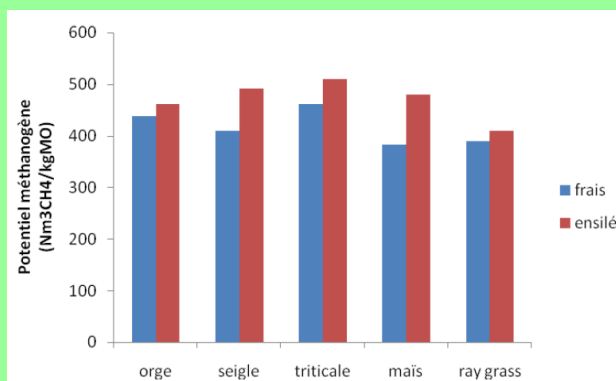
Illustration 121: Influence de l'ensilage sur la production de méthane (Lehtomäki 2006)
