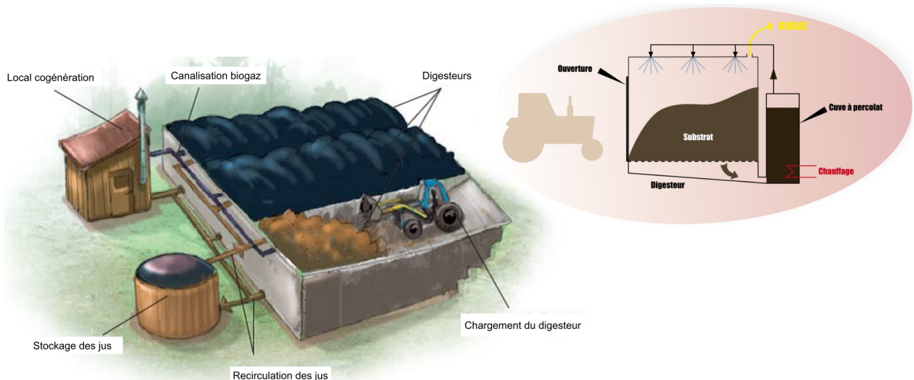
Illustration 92: Principe d'installation en voie sèche
