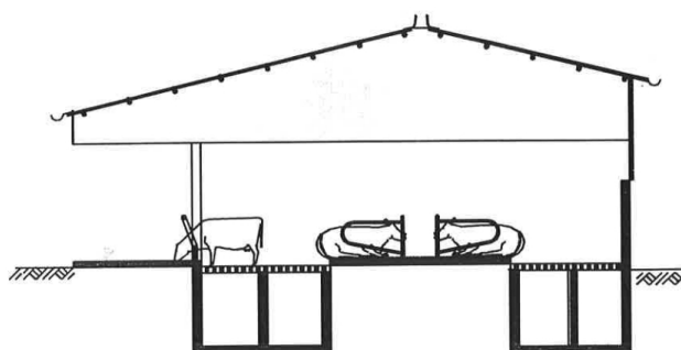
Illustration 53: Logette sur callebotis
