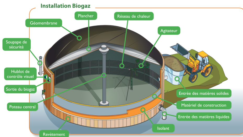
Illustration 90: Méthanisation par voie humide
