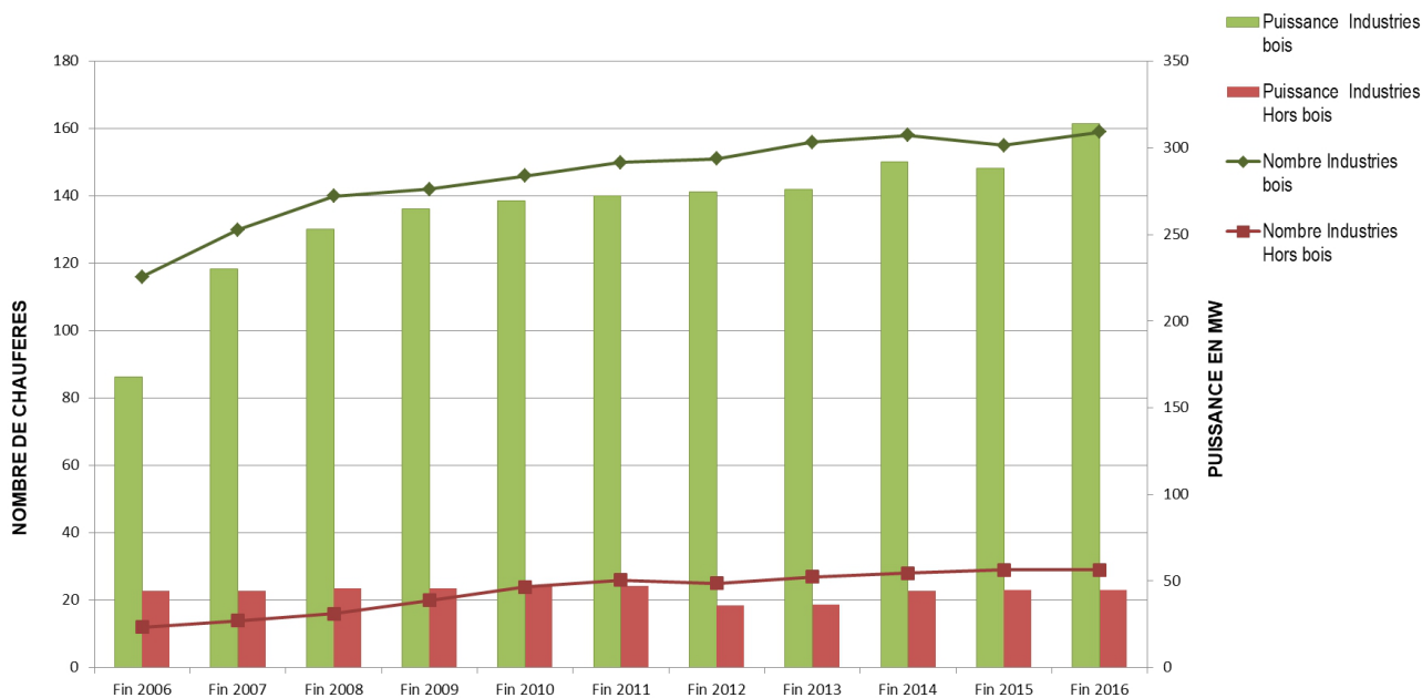
Illustration 86: Evolution Nombre/Puissance des chaufferies biomasse en BFC
