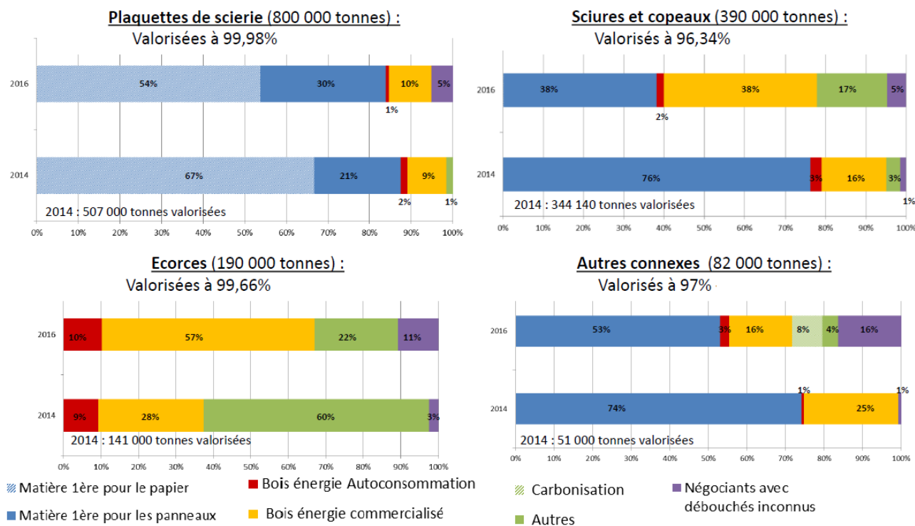
Illustration 50: Valorisation des connexes de scieries
